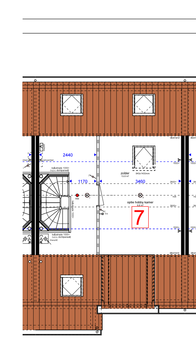
ZOLDER (optie 7)
