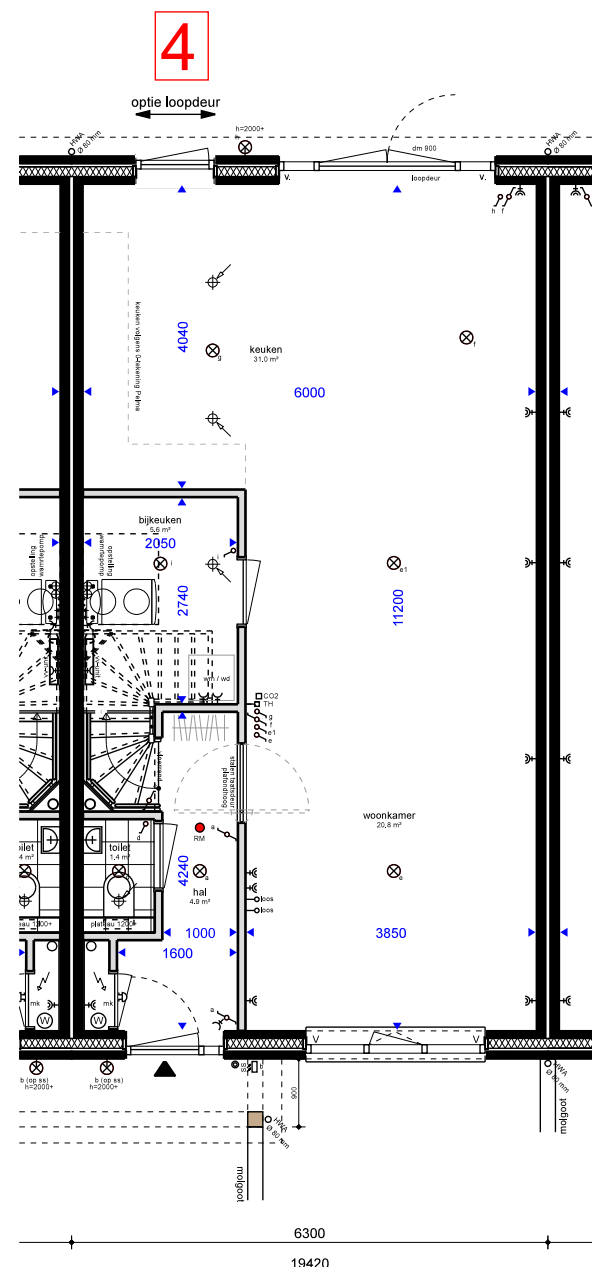
BEGANEGROND (optie 4)
