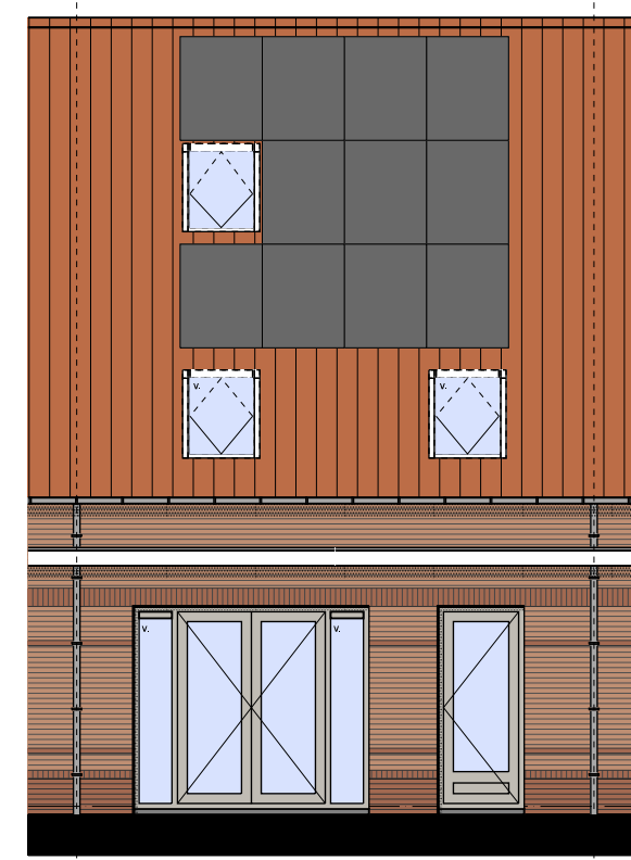
ACHTERGEVEL
