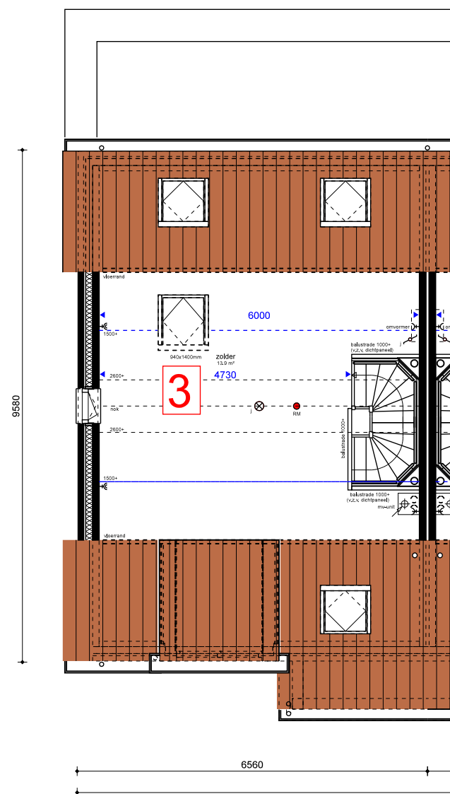
ZOLDER (optie 3)
