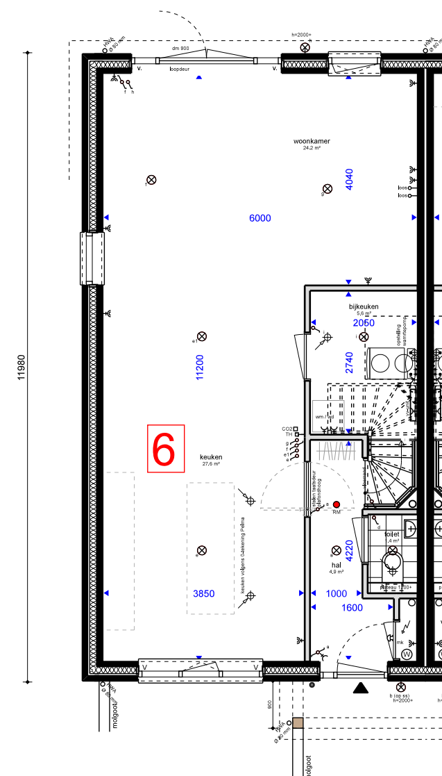
BEGANEGROND (optie 6)
