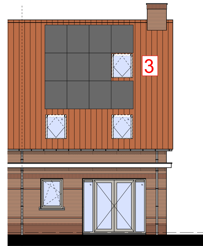
ACHTERGEVEL
