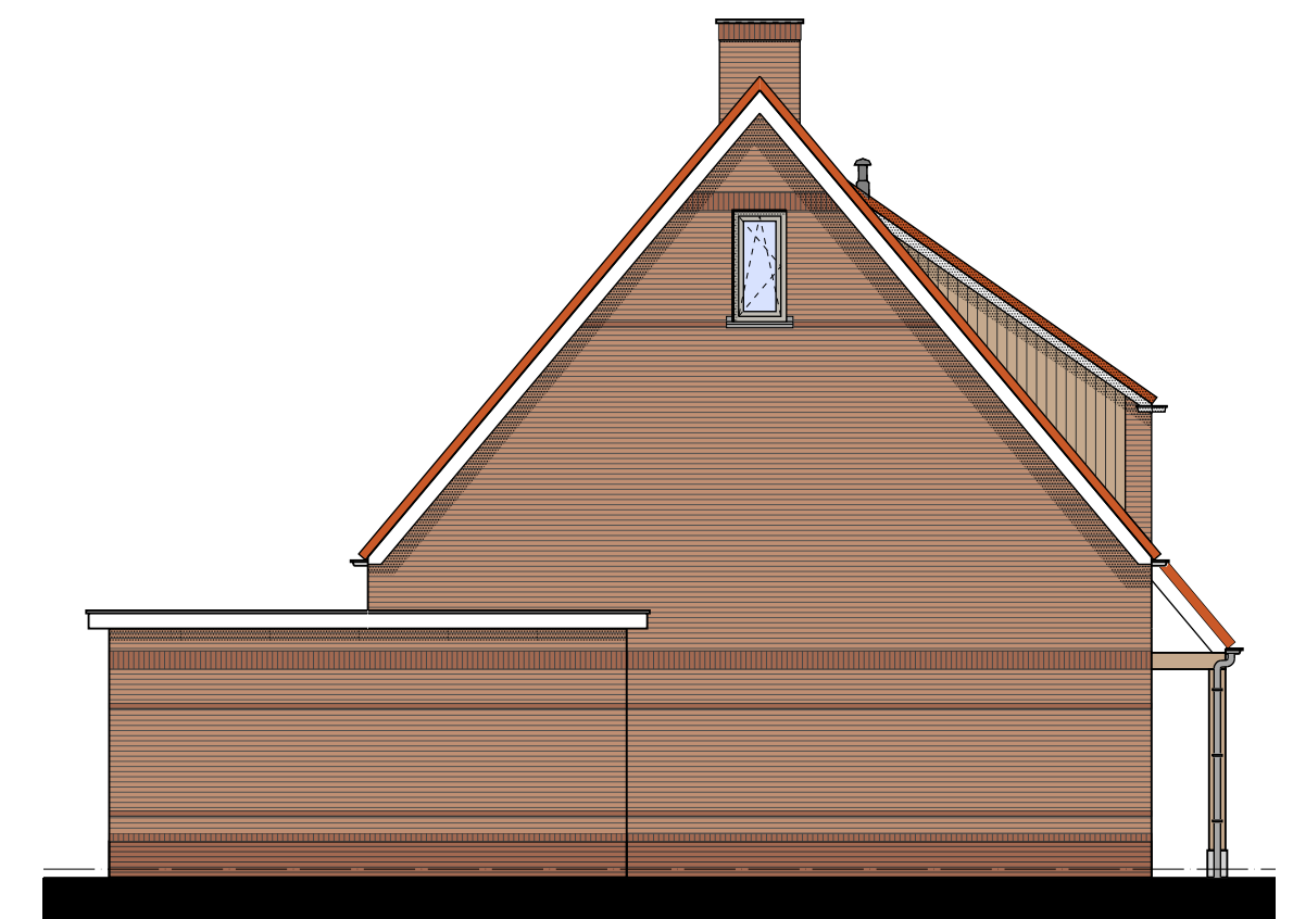
LINKERGEVEL
