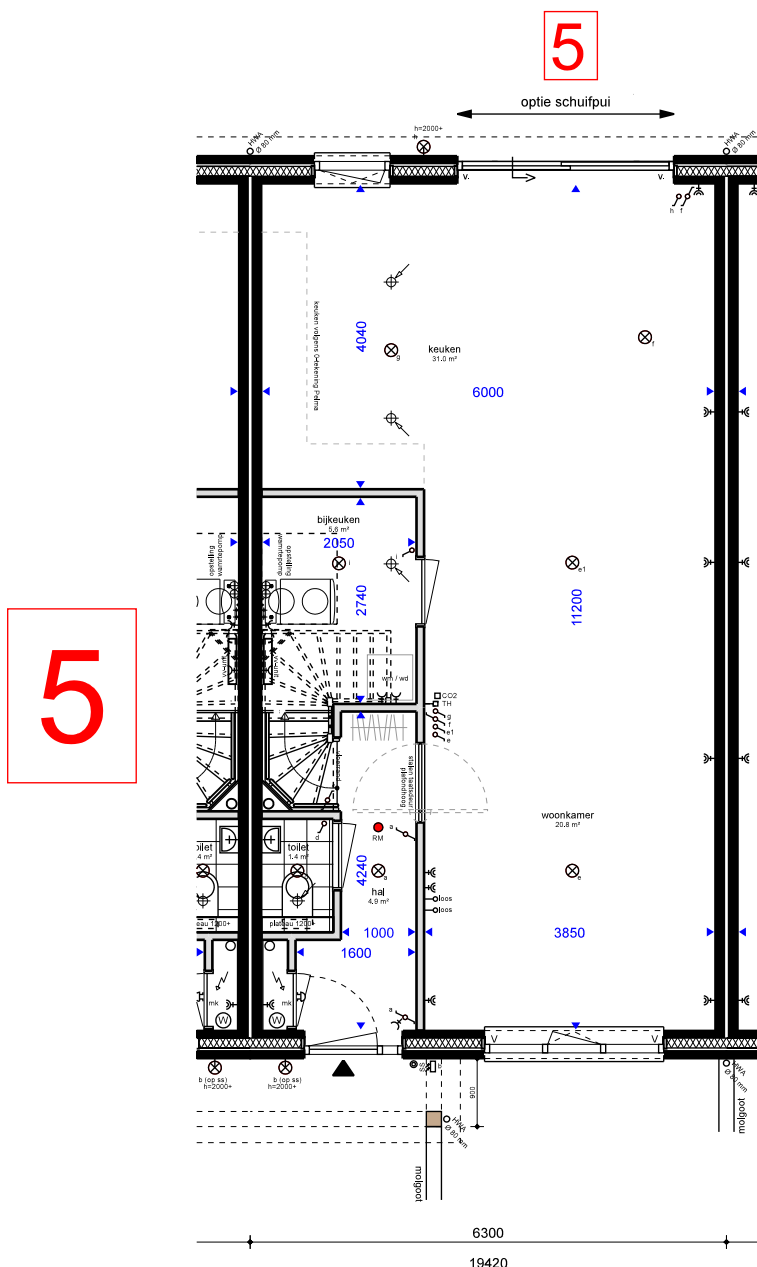
BEGANEGROND (optie 5)
